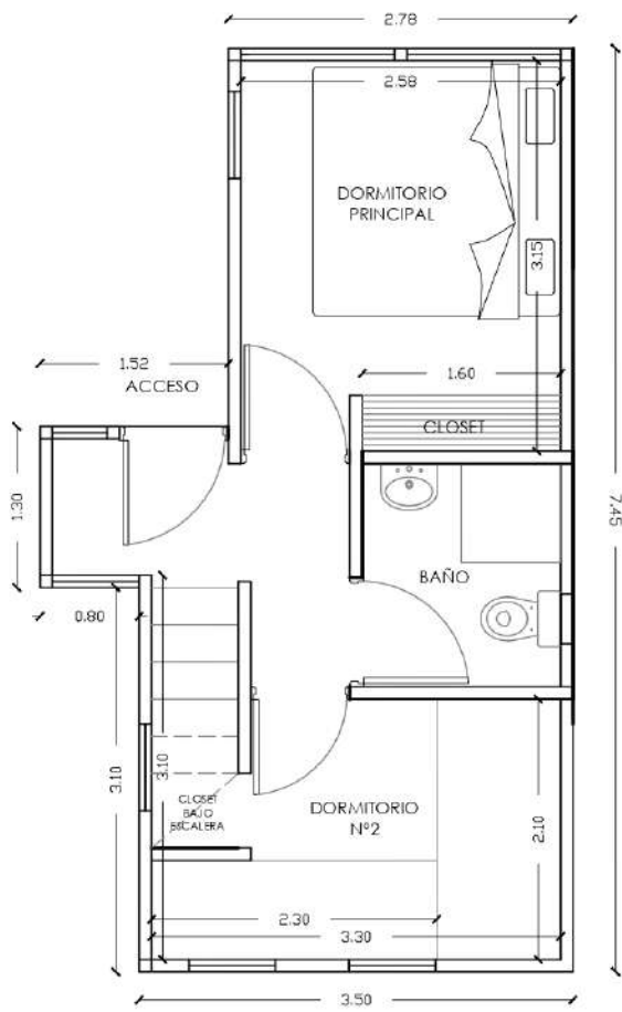
PLANTA ARQ 1º PISO
